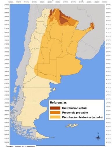
Situación del Yaguareté en Argentina.
